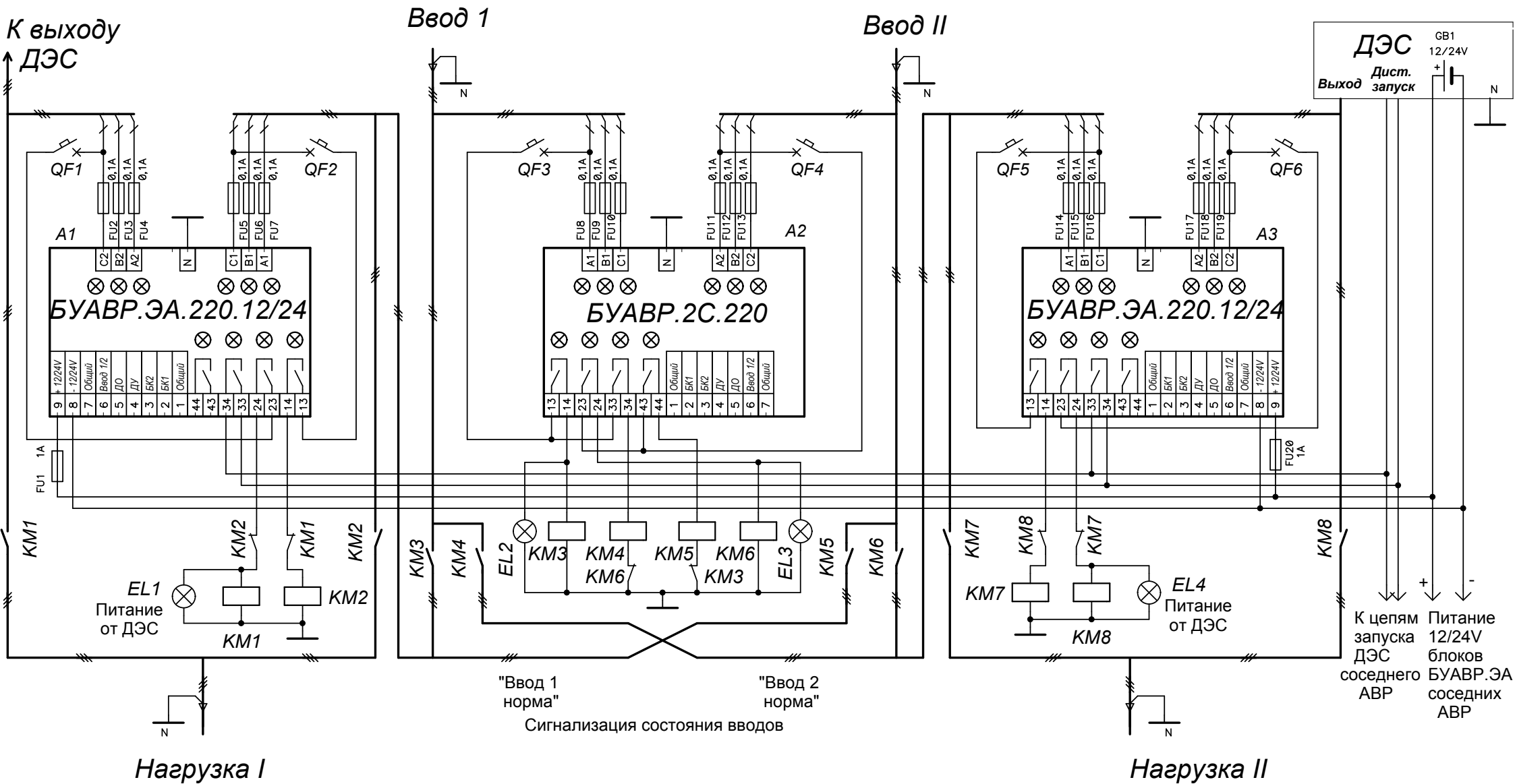
Схема АВР с 2 сетевыми вводами, ДЭС и двумя нагрузками, на контакторах, с управлением от БУАВР.2С и БУАВР.ЭА. В схеме предусмотрены: электрическая блокировка контакторов, сигнализация состояния сетевых вводов и сигнализация работы от ДЭС. QF1-QF6 - автоматические выключатели 1А, 1п отс.С(В) 6кА.
