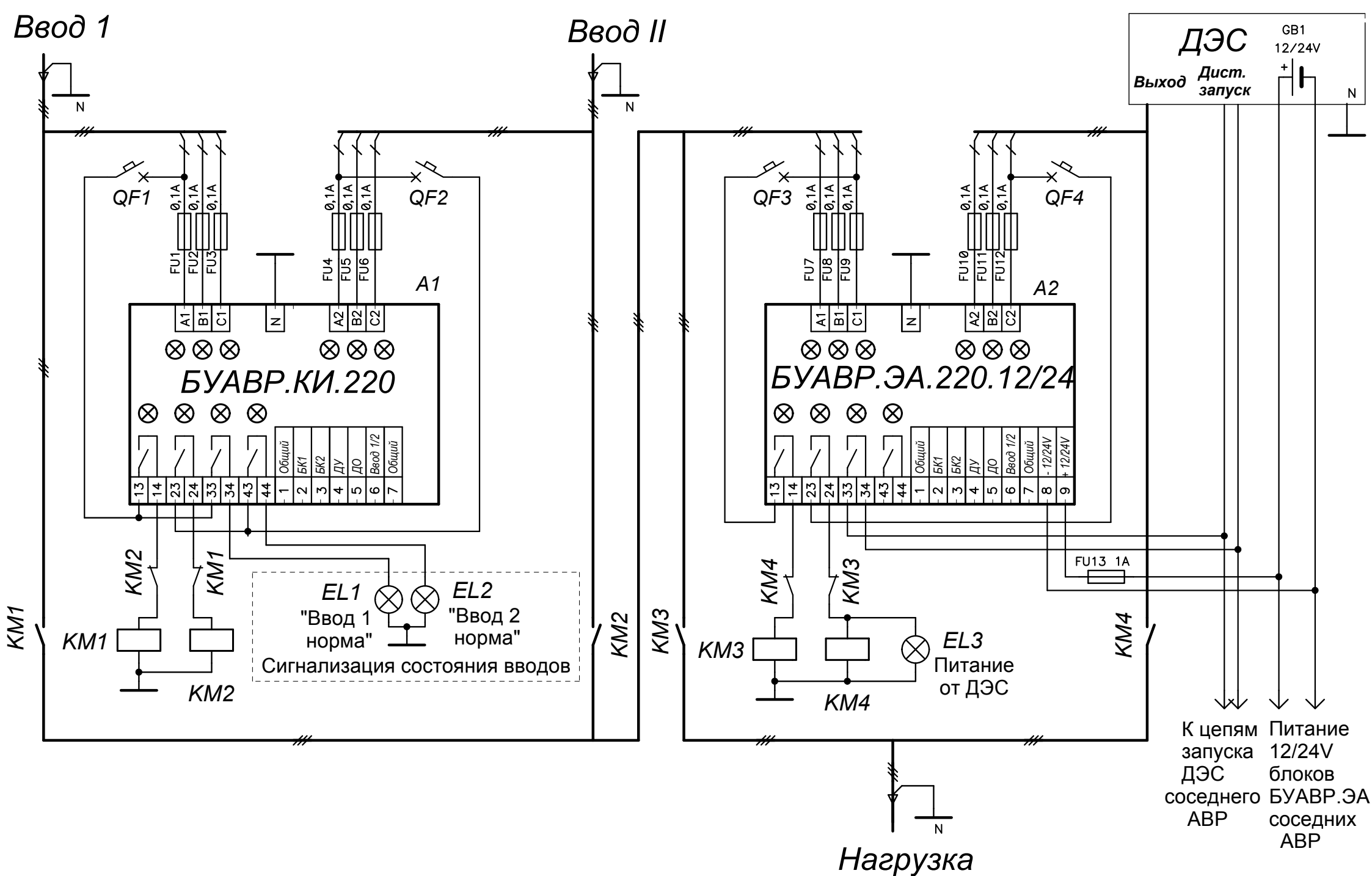
Схема АВР с 2 сетевыми вводами, ДЭС и одной нагрузкой, на контакторах, с управлением от БУАВР.КИ и БУАВР.ЭА. В схеме предусмотрены: электрическая блокировка контакторов, сигнализация состояния сетевых вводов и сигнализация работы от ДЭС. QF1-QF4 - автоматические выключатели 1А, 1п отс.С(В) 6кА.
