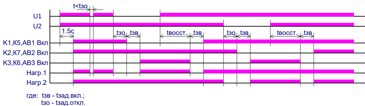
Рис. 4 Схема и временные диаграммы работы АВР на автоматических выключателях с мотор-приводом, двумя вводами, двумя группами равнозначных нагрузок, с секционным автоматическим выключателем с мотор-приводом, с электрической блокировкой секционного АВ, блокировкой АВ при срабатывании МТЗ и управлением от БУАВР.С.220.12/24.Т
